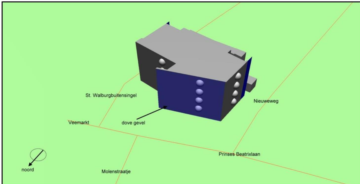
Figuur 9 3D-weergave locatie 'dove' gevel (zichthoek noordwest)
