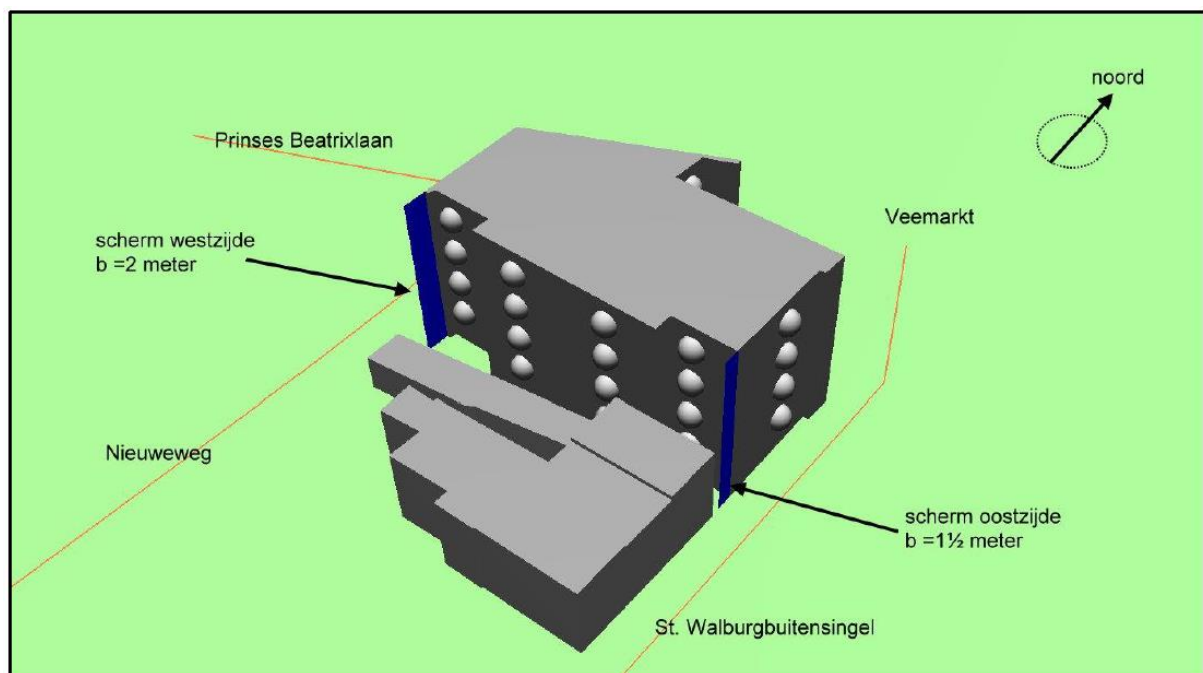
Figuur 8 3D-weergave locatie schermen (zichthoek zuidoost)
